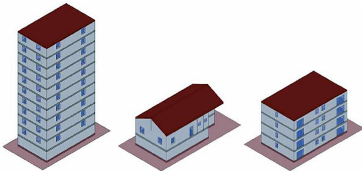
Fig. 4 - Gli edifici a diverso S/V posti a confronto [fonte: ricerca dell’Università Politecnica delle Marche (6)(7) ]. Da sinistra: edificio a torre, villetta, condominio.
