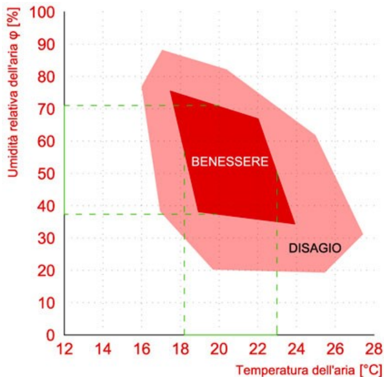
Fig. 3 - Diagramma del benessere termo-igrometrico, con individuazione delle condizioni di comfort e disagio, in relazione alla temperatura dell'aria (°C) e all'umidità relativa dell'aria (%).
