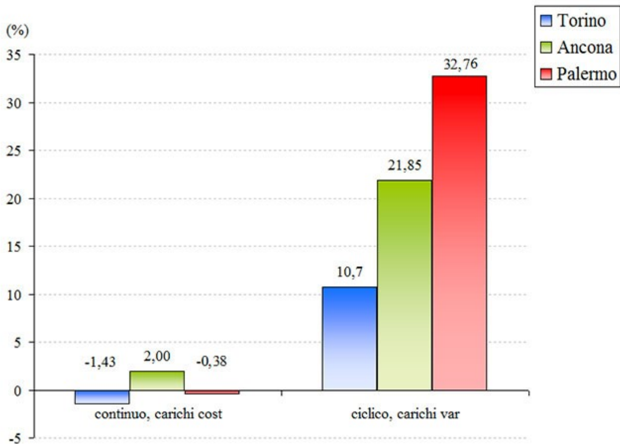
Fig. 5 - Incremento percentuale dei consumi per il riscaldamento invernale di edifici con struttura leggera rispetto a quelli con struttura massiva, in funzione delle ore di accensione dell'impianto e dei carichi interni, per l'edificio condominio posto a Palermo, Ancona, Torino [fonte: ricerca dell'Università Politecnica delle Marche(6)(7)].
