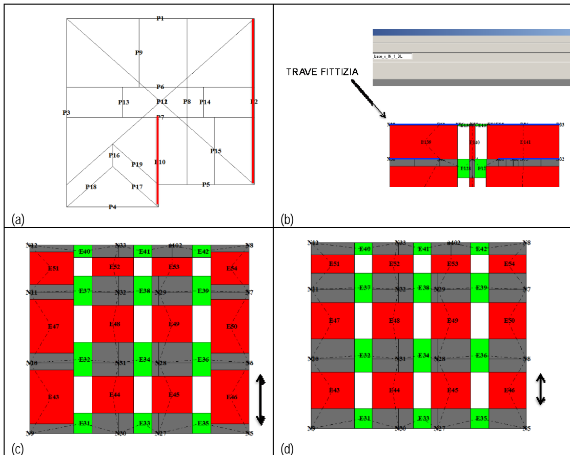
Fig. B-11. Modello strutturale a telaio equivalente (maschi in rosso; fasce in verde; nodi rigidi in grigio): (a) pianta con indicazione delle pareti illustrate; (b) in cui è stato considerato o meno l'effetto flangia in corrispondenza degli ammorsamenti; (c) due ipotesi assunte per la definizione della geometria del telaio equivalente: (c) Mesh-1 e (d) Mesh-2.
