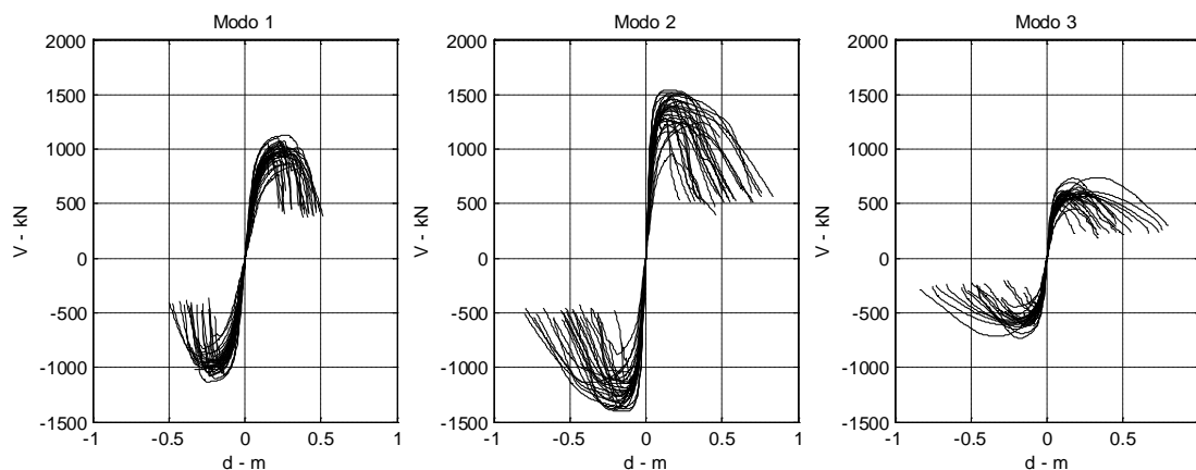
Fig. C-27 Modello C: Dispersione nelle curve di capacità per i tre modi significativi.
