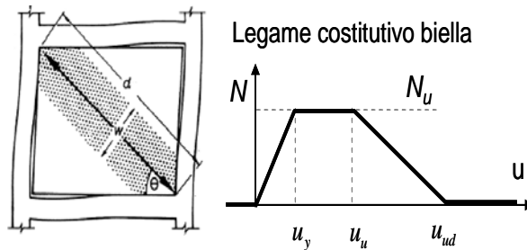
Fig. C-20 Legame costitutivo delle bielle equivalenti di tamponatura.
