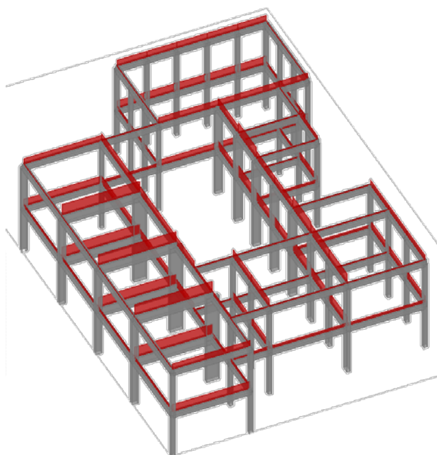
Fig. C-10 Modello preliminare e distribuzione dei carichi dei solai sulle travi.
