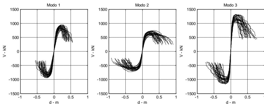
Fig. C-21 Modello A: Dispersione nelle curve di capacità per i tre modi significativi.
