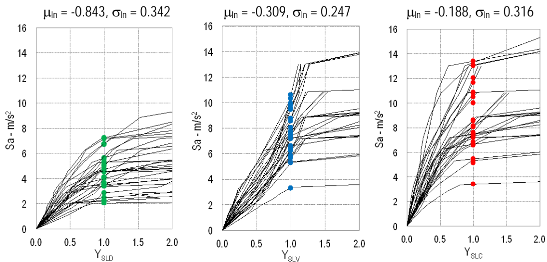
Fig. B-30 Curve di analisi dinamica incrementale in termini degli indicatori di stato limite Y_{SL} (in alto i parametri statistici della distribuzione lognormale dell'intensità che porta a SLD, SLV e SLC).
