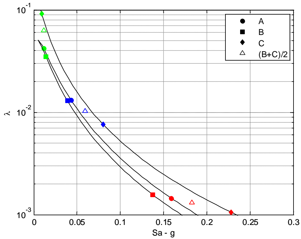
Fig. C-34 I risultati dei tre modelli a confronto: sono evidenziati anche i valori medi di B e C, media pesata dei rami equiprobabili dell'albero logico.
