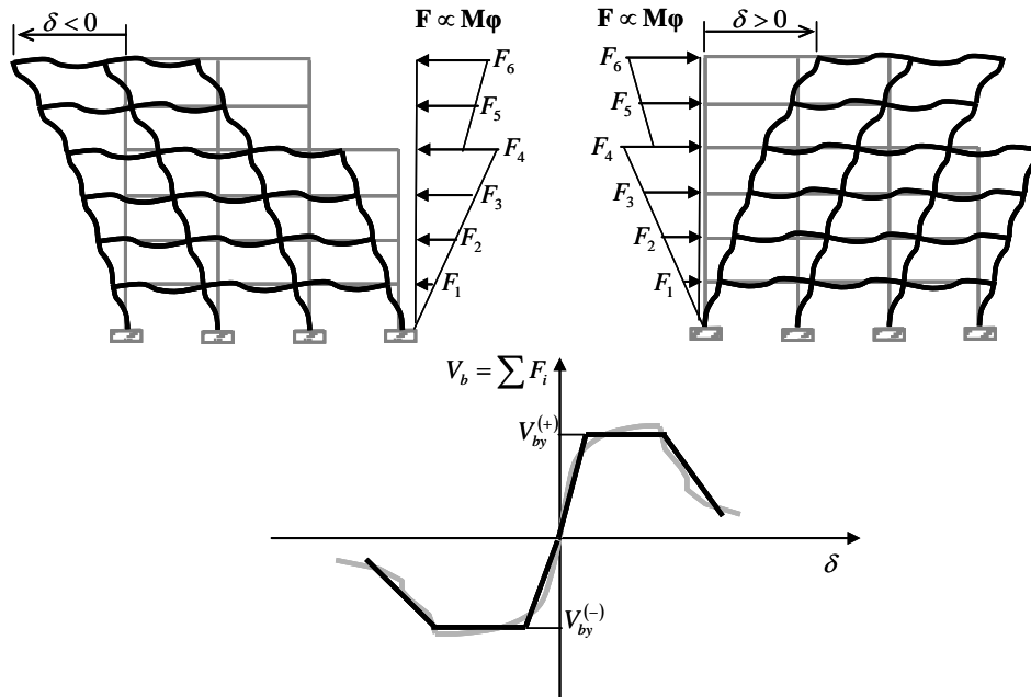
Fig. 2-4 Determinazione dell'involucro monotono del legame costitutivo dell'oscillatore equivalente nel caso generale di comportamento non simmetrico e modellazione con legami caratterizzati da degrado.
