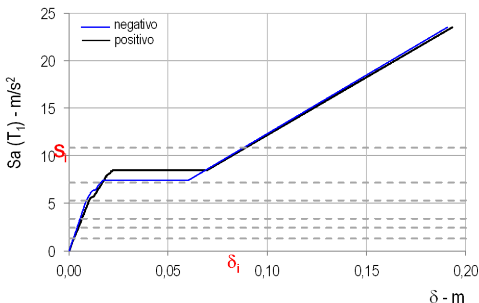
Fig. B-46 Curve ISA ottenute dal confronto tra la curva di capacità mediana e lo spettro di risposta mediano al variare del verso positivo e negativo (direzione X -Amm.1): le linee tratteggiate orizzontali esemplificano il potenziale utilizzo di tali curve al variare dei 6 valori di intensità sismica illustrati in Tabella B-18.
