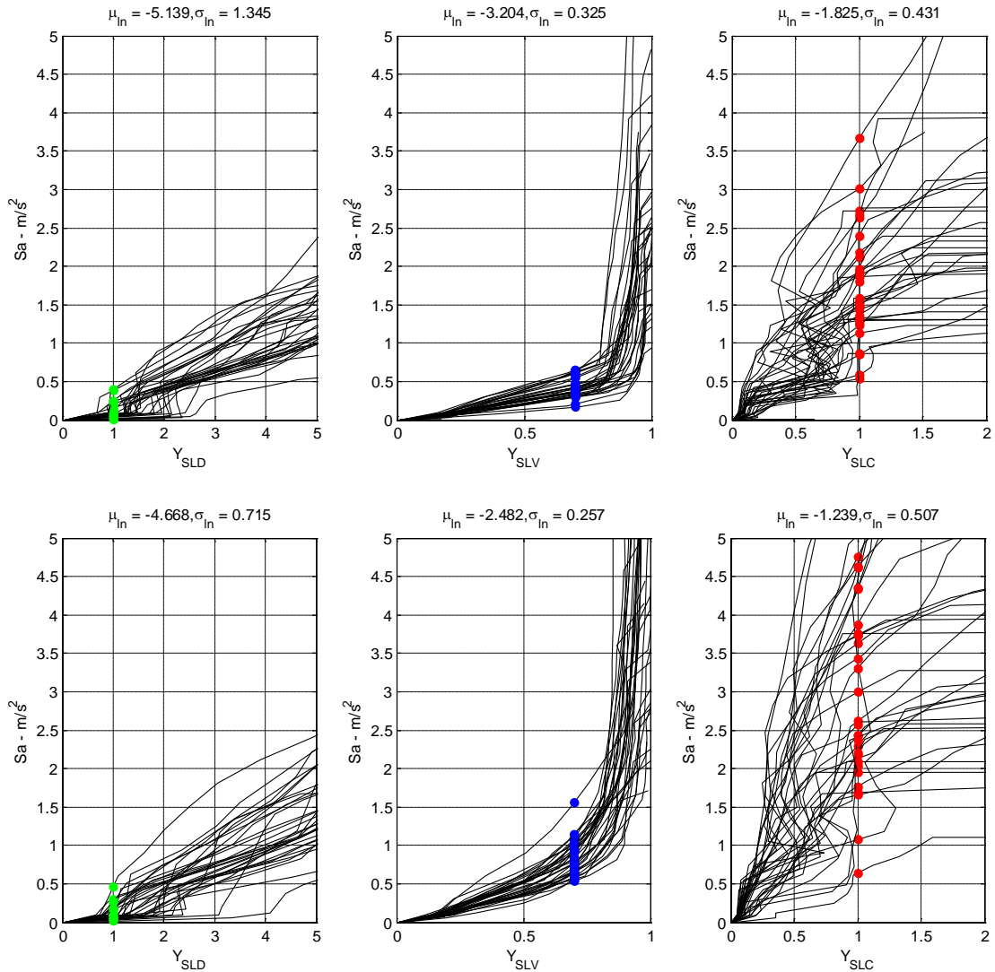
Fig. C-29 Modelli B (sopra) e C (sotto): Dettaglio delle curve di analisi dinamica incrementale, relazione intensità-indicatore di stato limite.
