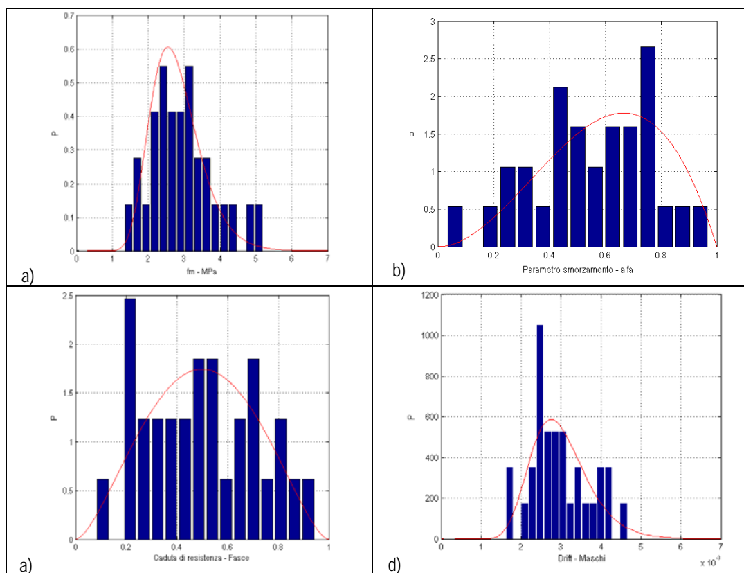
Fig. B-16 Istogrammi relativi ai 4 set di 30 parametri generati stocasticamente: a) resistenza a compressione della muratura f_m (dal gruppo 1); b) \alpha_{mT} relative alla risposta isteretica dei maschi (dal gruppo 8); c) \beta_{T3} (dal gruppo 7); \delta_{T3} (dal gruppo 6).
