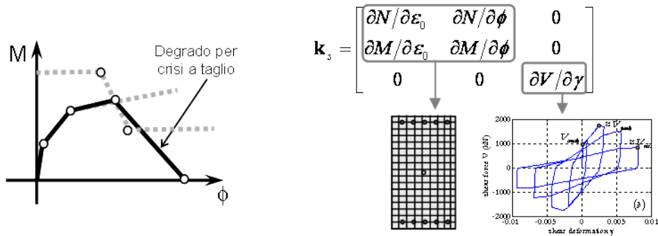
Fig. 4-4 Modelli di sezione diretti: alternative per la curva monotona (sinistra), effetto dell'interazione tra le sollecitazioni (destra).
