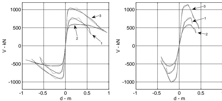
Fig. C-15 Curve di capacità e approssimazioni trilineari (modello senza degrado a sinistra, modello con degrado, destra). La tangente negativa nel modello con degrado è dovuta al contributo geometrico alla rigidità.
