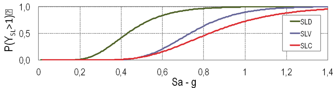
Fig. B-31 Curve di fragilità dei tre stati limite.
