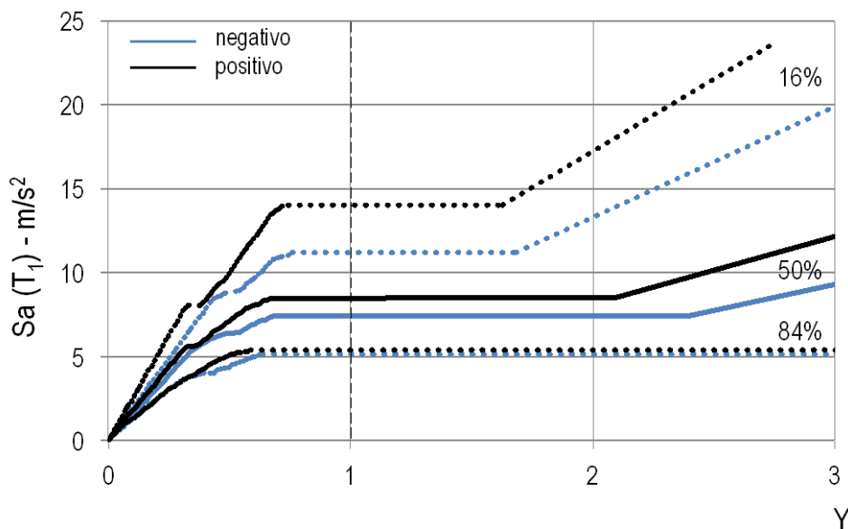
Fig. B-41 Curve ISA ottenute dal confronto tra la curva di capacità mediana e lo spettro di risposta mediano, al 16% e 84% percentile: Amm-1, direzione X (verso positivo e negativo) e SLC (che risulta in questo caso coincidente con lo SLV).
