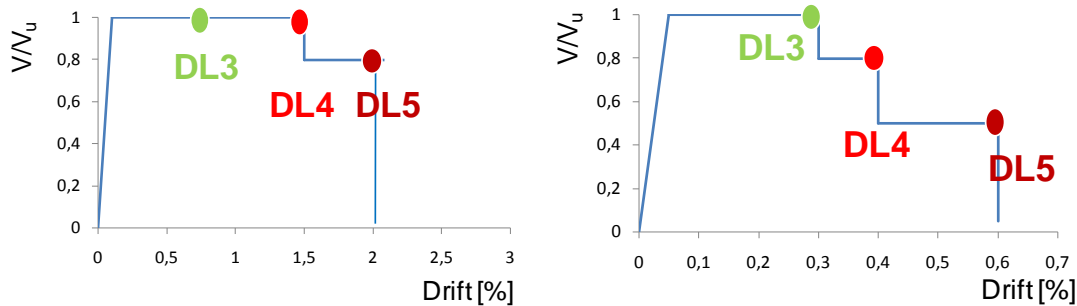
Fig. 3-2. Legami costitutivi taglio-drift per maschi murari: a) rottura a pressoflessione, b) rottura a taglio.
