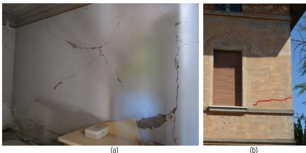
(a) (b) Fig. B-3 Lesioni nei maschi: (a) rottura a taglio in una parete interna; (b) pressoflessione in un maschio poco caricato al secondo piano di una parete perimetrale.
