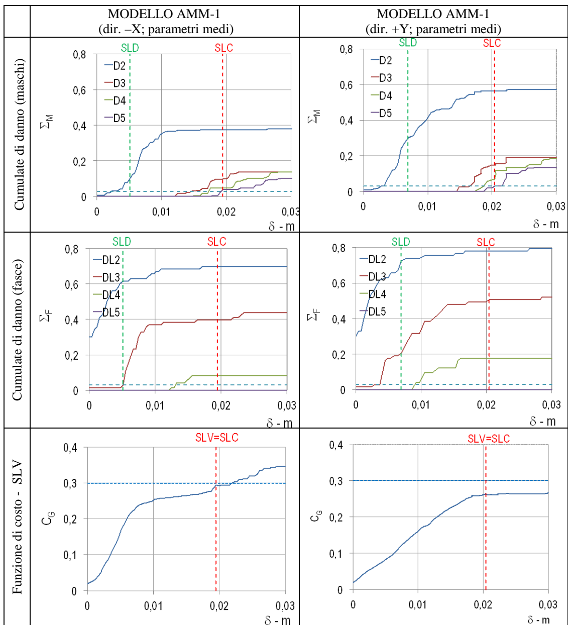
Fig. B-38 Evoluzione delle cumulate del danno e della variabile del costo di riparazione globale
