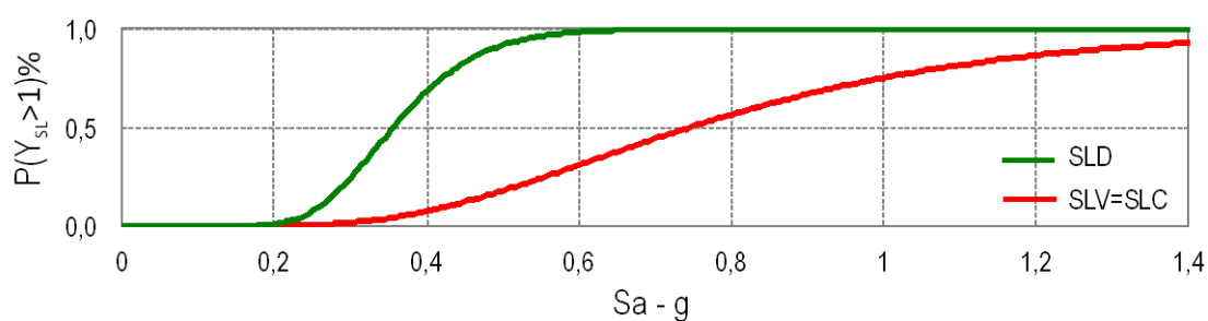
Fig. B-43 Curve di fragilità per i tre stati limite, ottenute per il primo ramo dell'albero logico (Amm-1).
