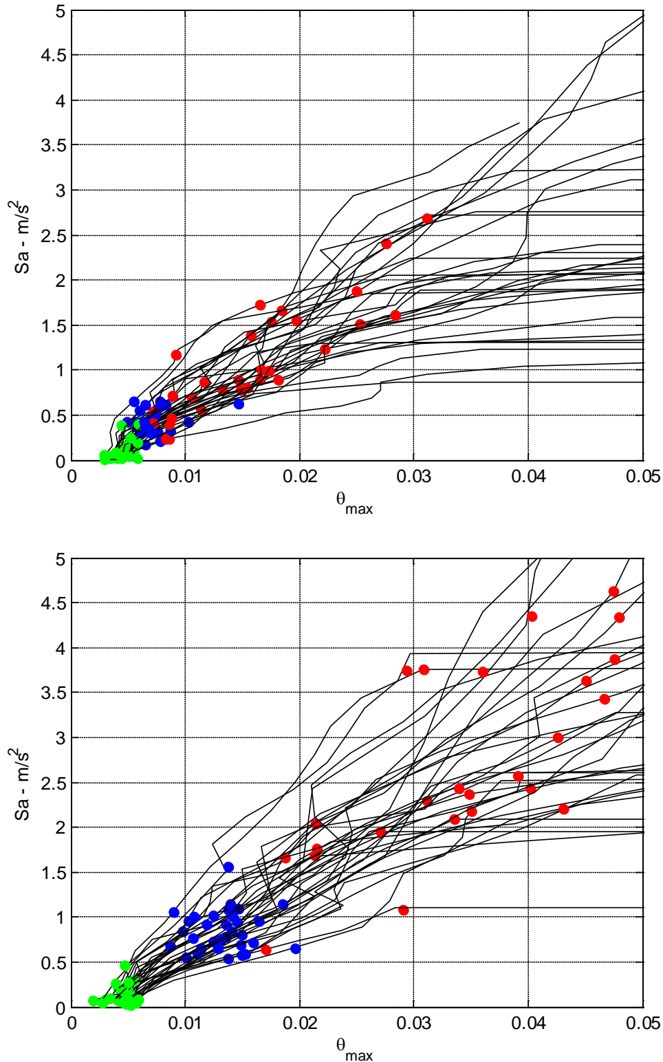
Fig. C-28 Modelli B (sopra) e C (sotto): Curve di analisi dinamica incrementale della struttura (combinazione delle curve modali, vedi Fig. C-16).
