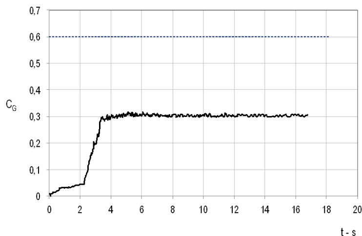
Fig. B-26 Andamento nel tempo dei parametri necessari al calcolo degli indicatori di stato limite alla scala dell'elemento (cumulata del danno \Sigma_{SLD} e funzione di costo C_G ), risultanti dall'applicazione della registrazione 1 scalata al valore S_a(T_1)=6.25 \text{ m/s}^2 .
