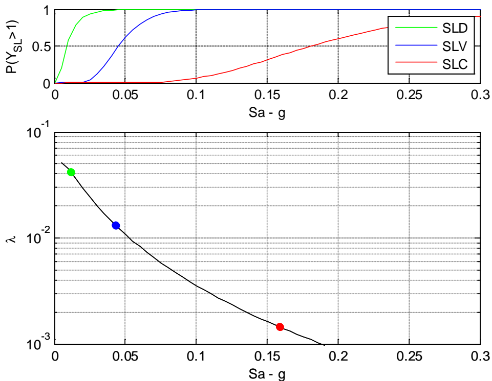
Fig. C-25 Modello A: Curve di fragilità (in alto), e curva di pericolosità per S_a(T_1 = 1.42s) (in basso), con indicazione dei valori delle frequenze medie annue di superamento per i tre SL.
