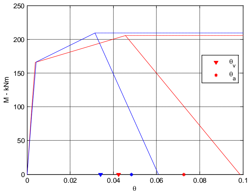
Fig. C-14 Errore dei modelli: legame costitutivo M-\theta relativo a un elemento con valori medi delle variabili aleatorie (blu) e per uno dei campionamenti (rosso).
