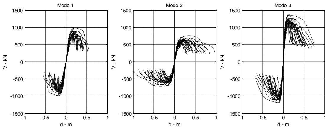
Fig. C-26 Modello B: Dispersione nelle curve di capacità per i tre modi significativi.
