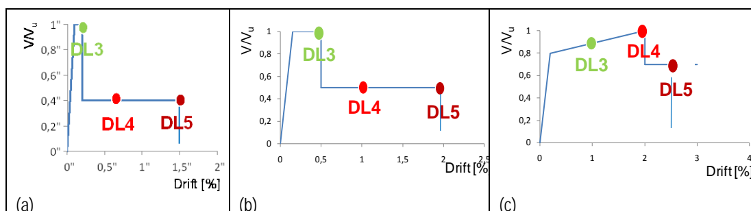
Fig. 3-3. Legami costitutivi taglio-drift per fasce murarie: a) fascia sorretta da arco in muratura; b) architrave in legno, acciaio o c.a.; c) architrave accoppiato ad elemento resistente a trazione.
