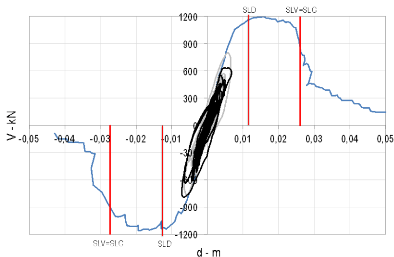
Fig. B-20 Direzione Y: confronto tra i risultati delle analisi non lineari statiche e dinamiche
