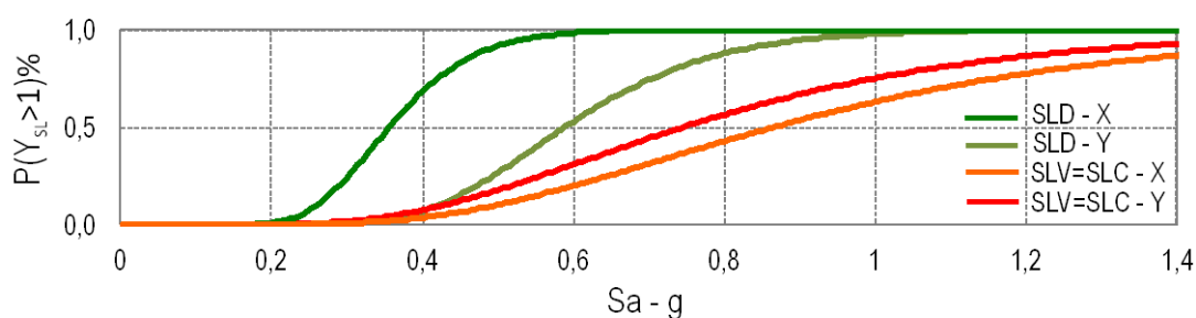
Fig. B-42 Curve di fragilità per i tre stati limite, ottenute per il primo ramo dell'albero logico, considerando la risposta nelle due direzioni X e Y.
