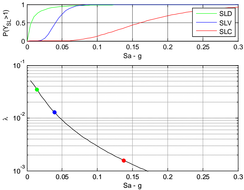
Fig. C-30 Modello B: Curve di fragilità (in alto), e curva di pericolosità per S_a ( T_1 = 1.53s ) (in basso), con indicazione dei valori delle frequenze medie annue di superamento per i tre SL.
