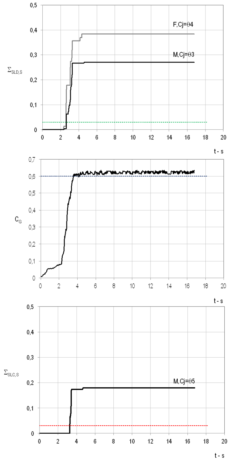
Fig. B-27 Andamento nel tempo dei parametri necessari al calcolo degli indicatori di stato limite alla scala dell'elemento (cumulate del danno \Sigma_{SLD} , \Sigma_{SLC} e funzione di costo C_G ), risultanti dall'applicazione della registrazione 1 scalata al valore S_a(T_1)=10.84 \text{ m/s}^2 .
