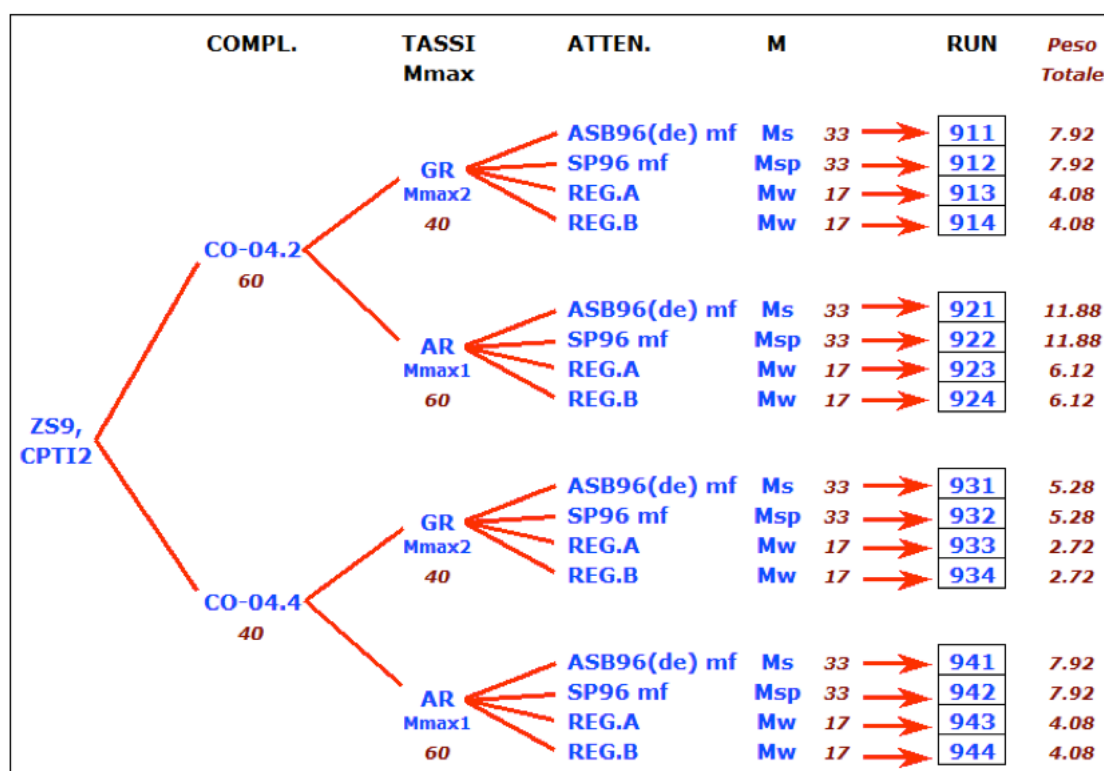
Fig. A-3 Albero logico utilizzato in (INGV, 2004) per determinare la distribuzione dell'accelerazione di picco al suolo.
