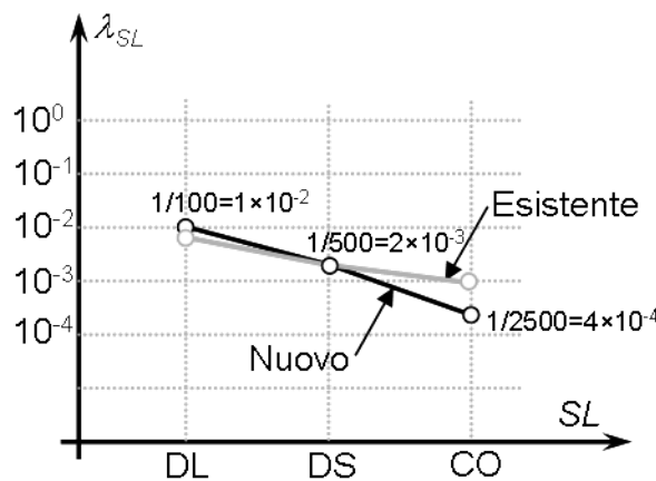
Fig. A-2 Variazione della frequenza media annua di superamento degli SL per edifici nuovi ed esistenti.
