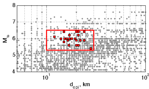
Fig. C-6 Coppie magnitudo-distanza delle registrazioni della base dati ( 5 \text{ km} < R < 100 \text{ km} ). Sono evidenziate le coppie relative alle registrazioni selezionate e gli estremi degli intervalli obiettivo.
