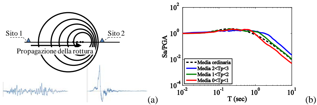
Fig. A-5 (a) Rappresentazione semplificata degli effetti impulsivi della direttività ed esempio in relazione al terremoto di Landers in California (1992). (b) Spettri elastici medi di accelerazione nel caso di segnali impulsivi ed ordinari; tutti gli spettri sono adimensionalizzati per i valori dell'accelerazione di picco al suolo ( peak ground acceleration o PGA). Si noti la differenza sistematica intorno al periodo dell'impulso.
