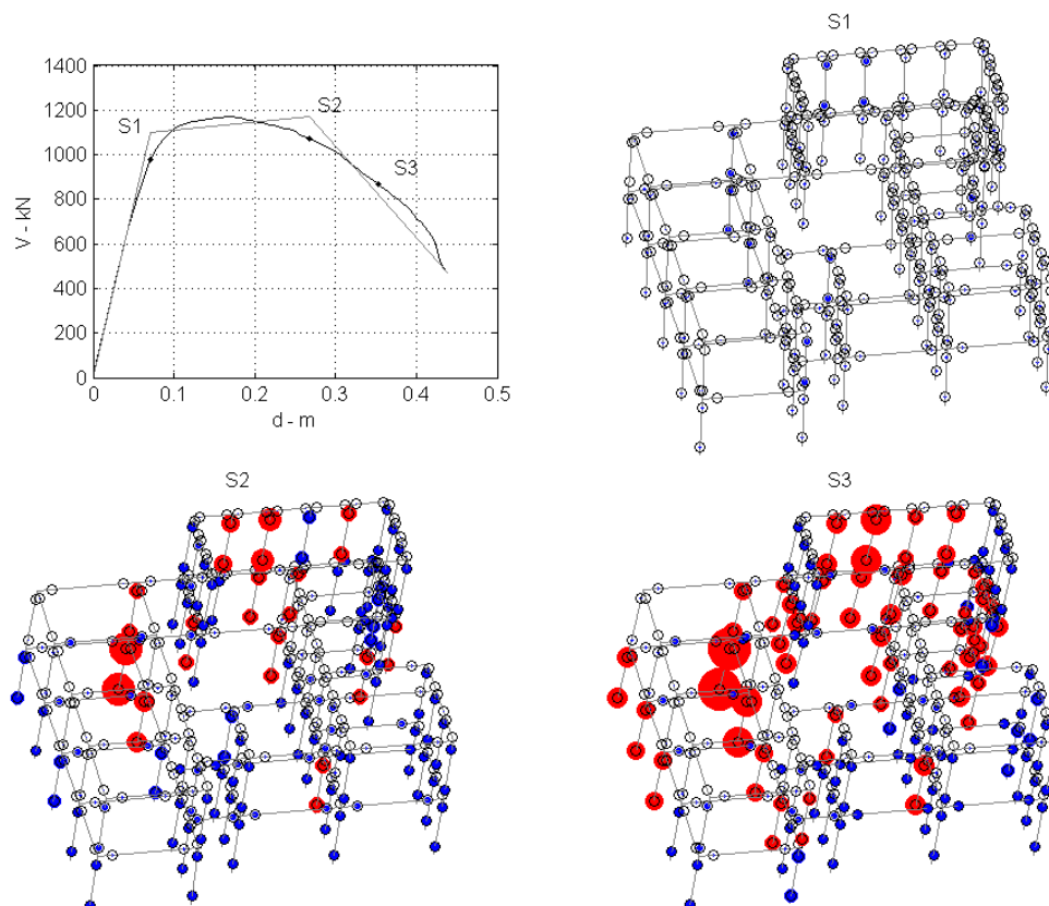
Fig. C-32 Curva di capacità e deformate corrispondenti ai tre punti: snervamento, picco e intermedio sul ramo di degrado.
