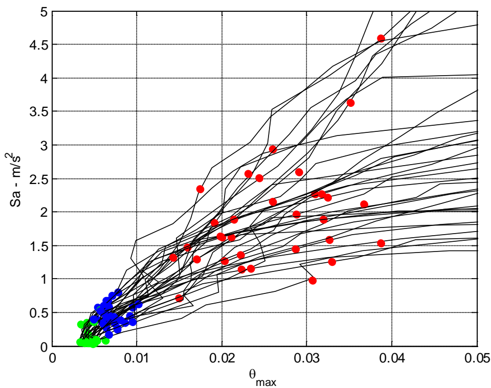
Fig. C-23 Modello A: Curve di analisi dinamica incrementale della struttura (combinazione delle curve modali, vedi Fig. C-16).
