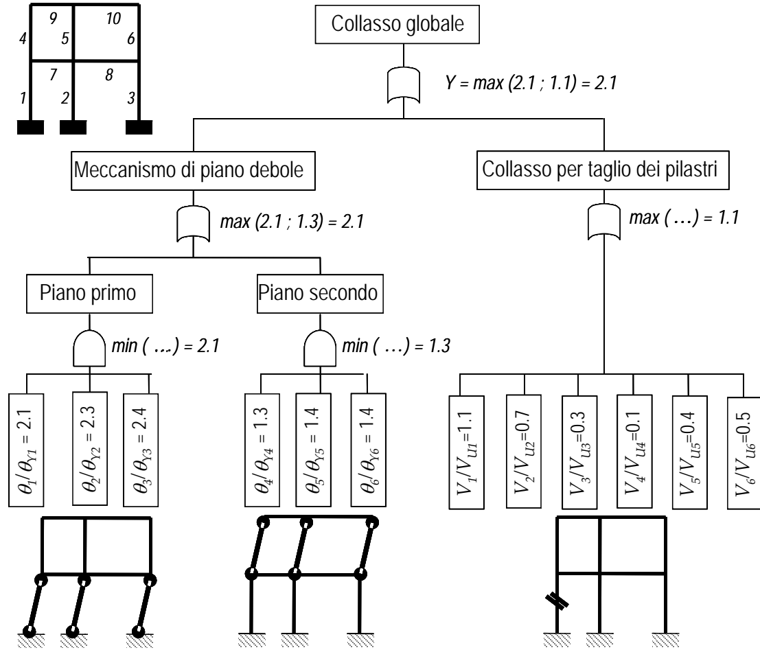
Fig. A-6 Rappresentazione della crisi della struttura come combinazione di sotto-sistemi (meccanismi) alternativi.
