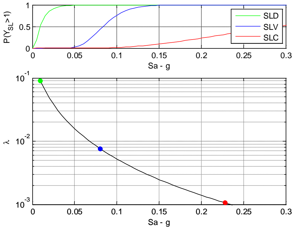
Fig. C-31 Modello C: Curve di fragilità (in alto), e curva di pericolosità per S_a ( T_1 = 1.18s ) (in basso), con indicazione dei valori delle frequenze medie annue di superamento per i tre SL.
