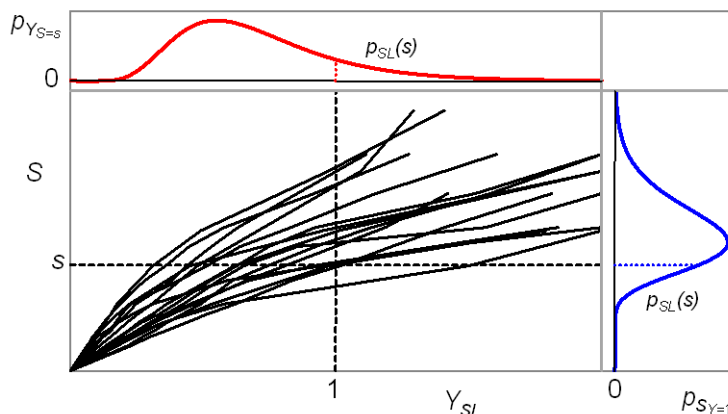
Fig. A-7 Valutazione della fragilità a partire dalle curve IDA (o ISA) attraverso le (2.14) e (A.12).
