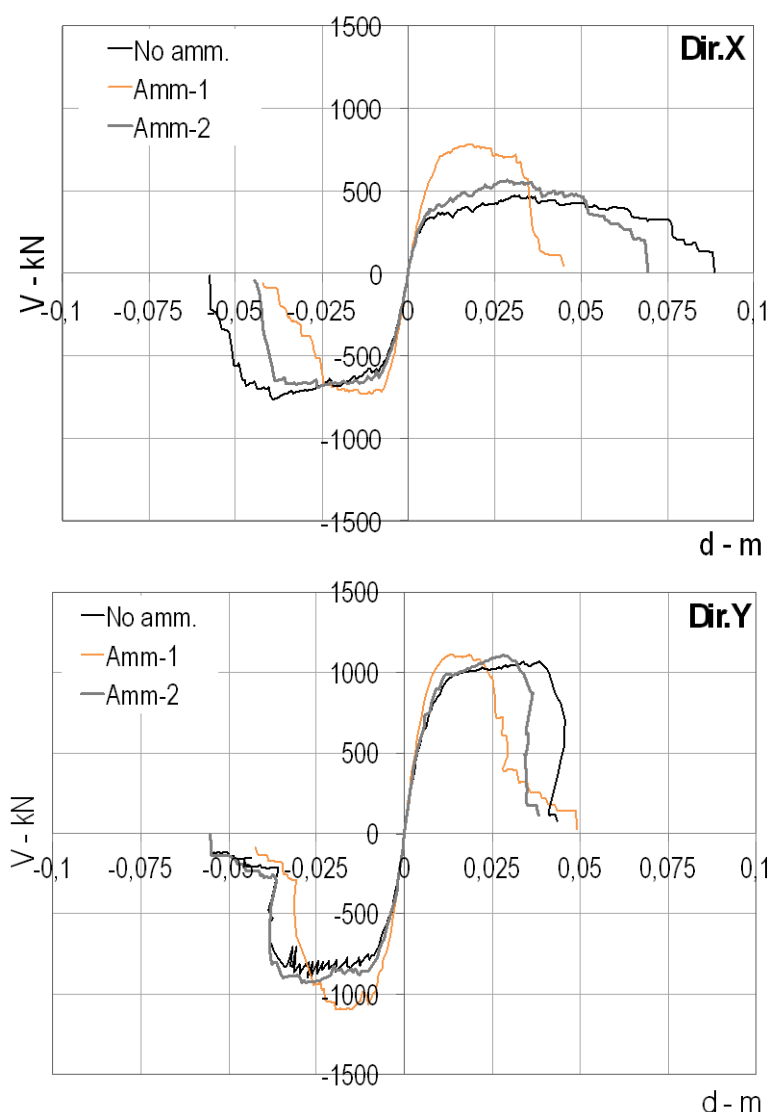
Fig. B-13 Curve pushover risultanti in direzione X e Y (verso positivo e negativo) al variare delle due ipotesi di ammorsamento (Amm-1 e Amm-2) e nel caso di assenza di ammorsamento
