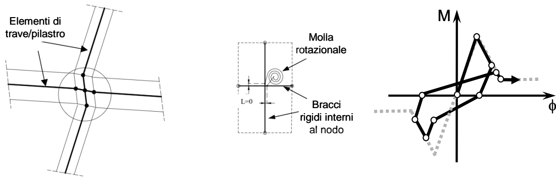
Fig. 4-7 Modello di risposta dei nodi esterni: geometria (sinistra), legame costitutivo (destra).
