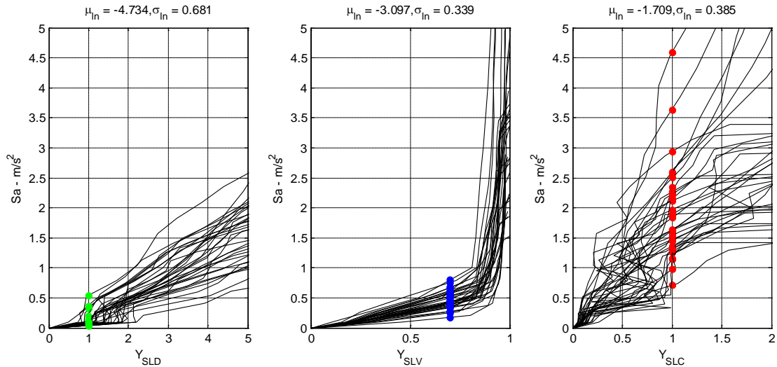
Fig. C-24 Modello A: Dettaglio delle curve di analisi dinamica incrementale, relazione intensità-indicatore di stato limite.
