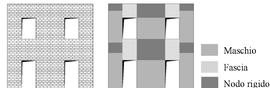
Fig. 3-1. Idealizzazione attraverso il telaio equivalente di una parete in muratura
