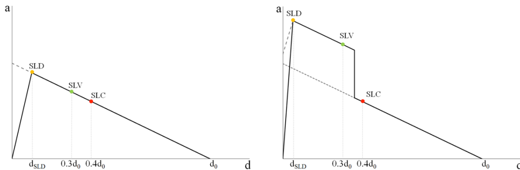
Fig. 3-4. Spostamenti sulla curva di capacità dei meccanismi locali corrispondenti al raggiungimento dei diversi stati limite: a) cinematismo senza elementi resistenti elasto-plastici; b) cinematismo con elementi resistenti elasto-plastici (catene).
