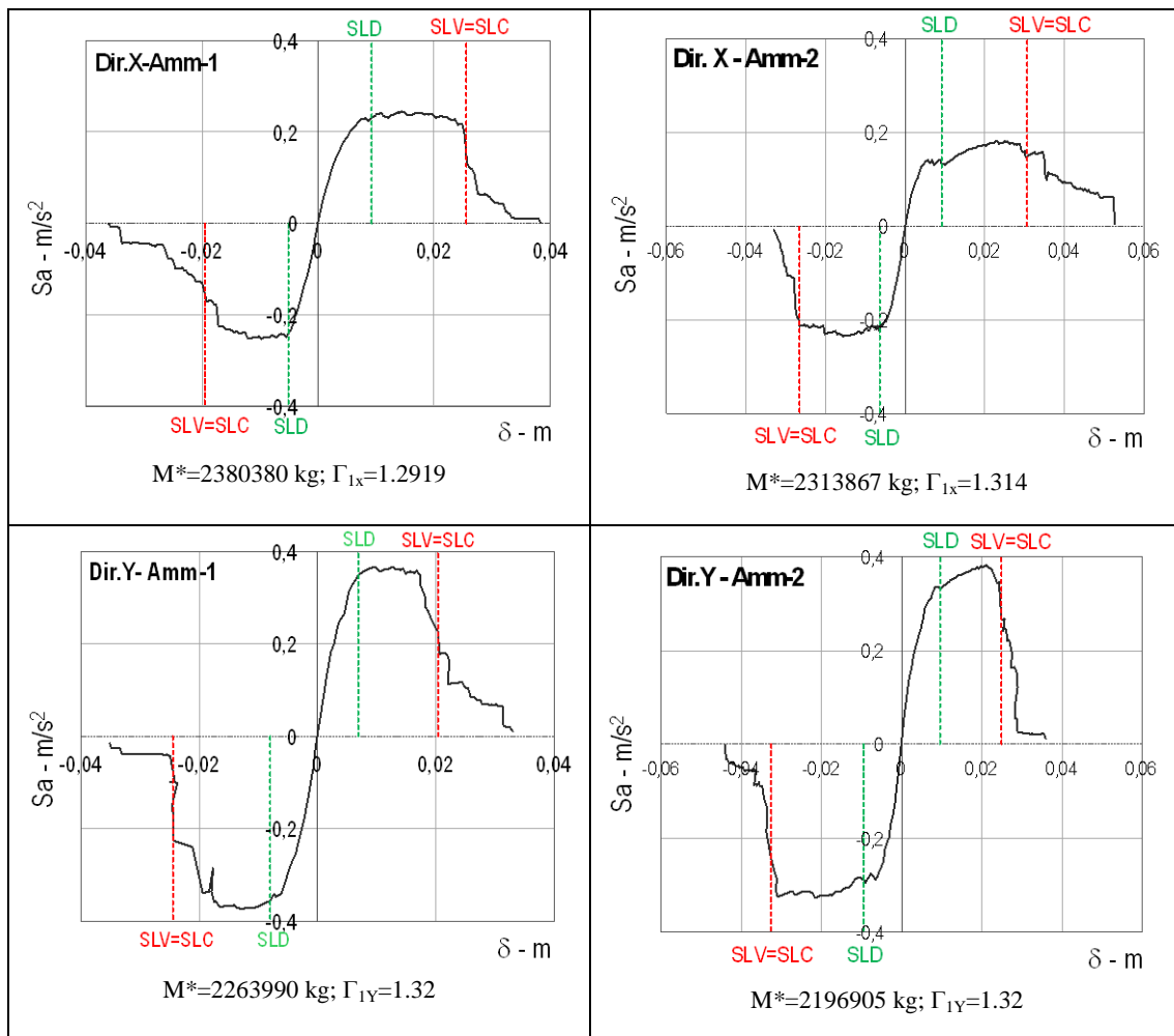
Fig. B-35 Risultati delle analisi statiche non lineari in termini di curva di capacità (conversione nell'oscillatore equivalente): direzione X verso positivo e negativo per i due rami dell'albero logico (valori medi per tutte le variabili aleatorie)
