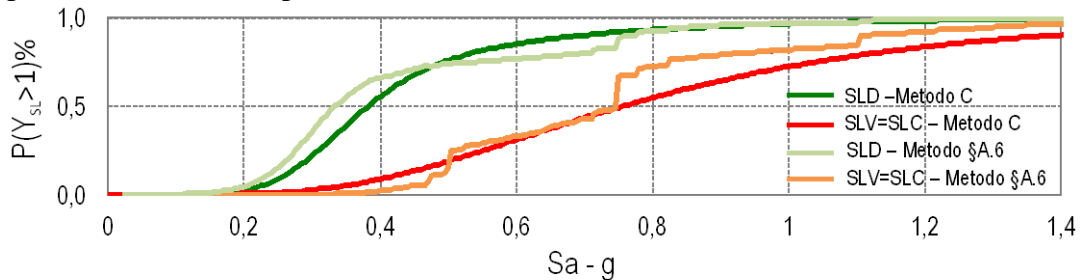
Fig. B-52 Curve di fragilità finali per i tre stati limite a confronto come ottenute dal Metodo C e dal metodo illustrato in §A.6 (dalla combinazione dei rami dell'albero logico)
