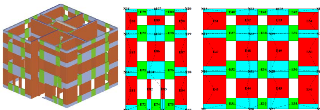
Fig. B-8 Modello strutturale tridimensionale e mesh a telaio equivalente di due prospetti.
